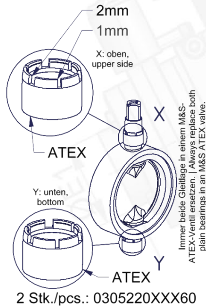
Bild 17 SV04 Dichtung und Klappe mit leitfähigen Gleitlagern
