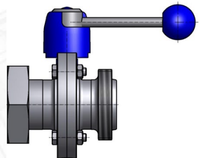
Bild 6 Scheibenventil SV04 KG IDF/DS/RJT/SMS Art.-Nr.: 56544/56554/56564/56474
