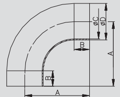
Schweißbogen DIN 11852-BL 90° welding bend DIN 11852-BL 90°
